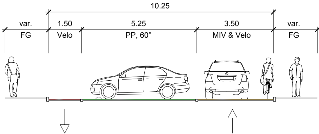
Querschnitt "Schrägparkierung"
