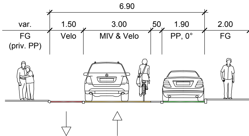
Querschnitt "Längsparkierung"
